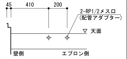
カウンター水栓 取付部詳細
