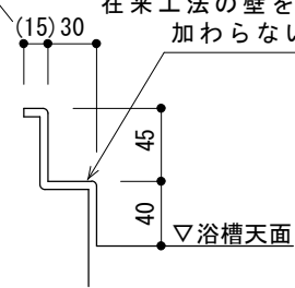
壁載り (防水リム) 部詳細 S=1/5
