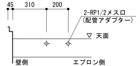
カウンター水栓 取付部詳細
