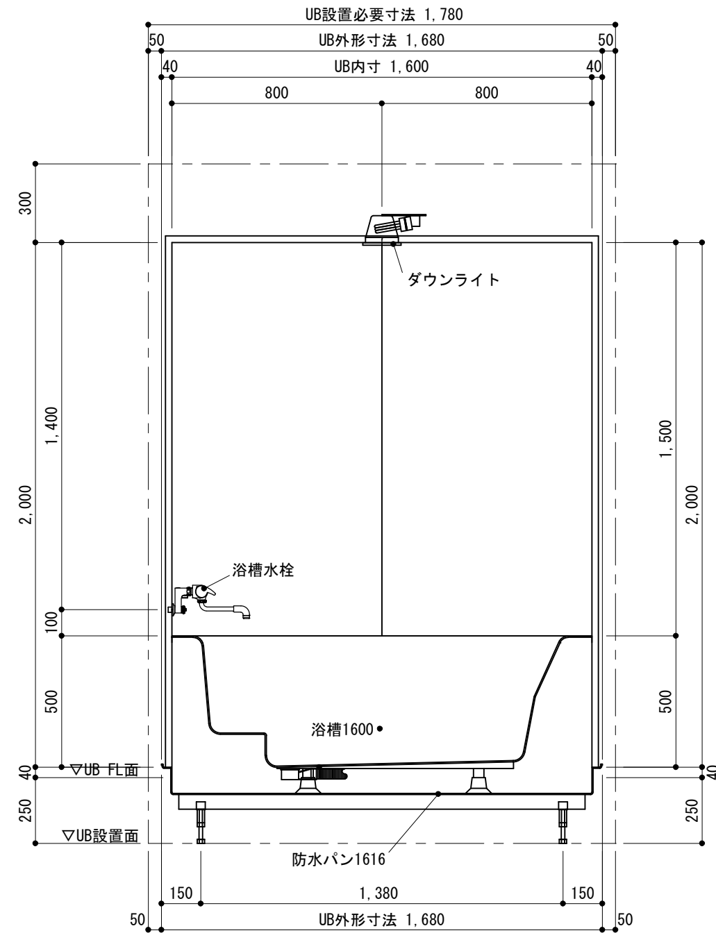
D展開図
