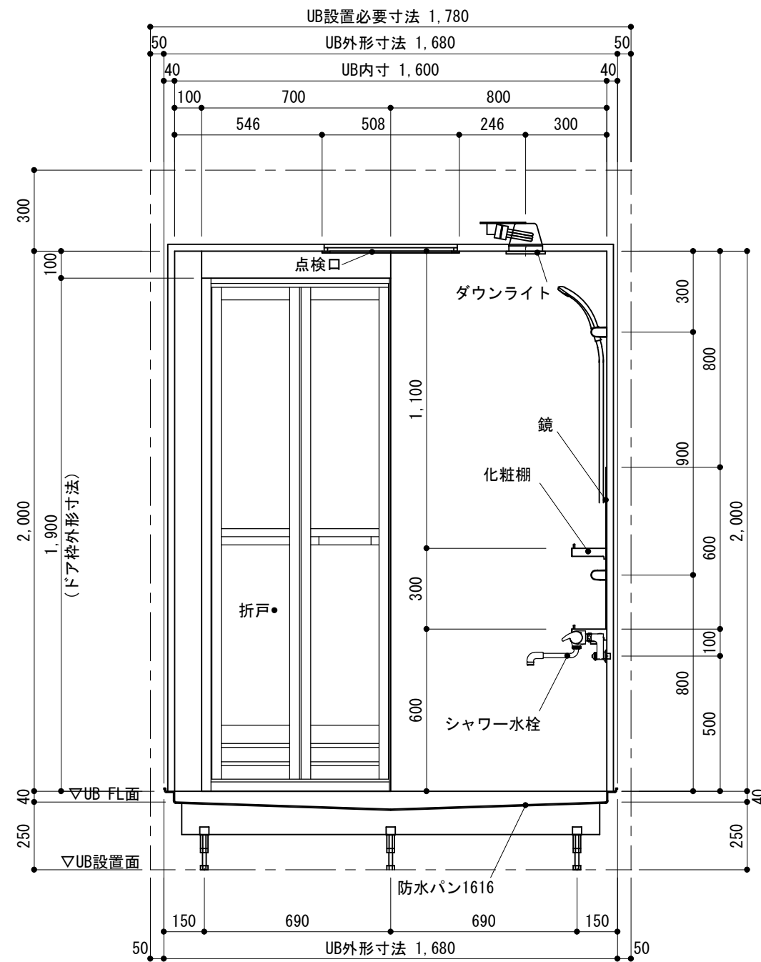
B展開図
