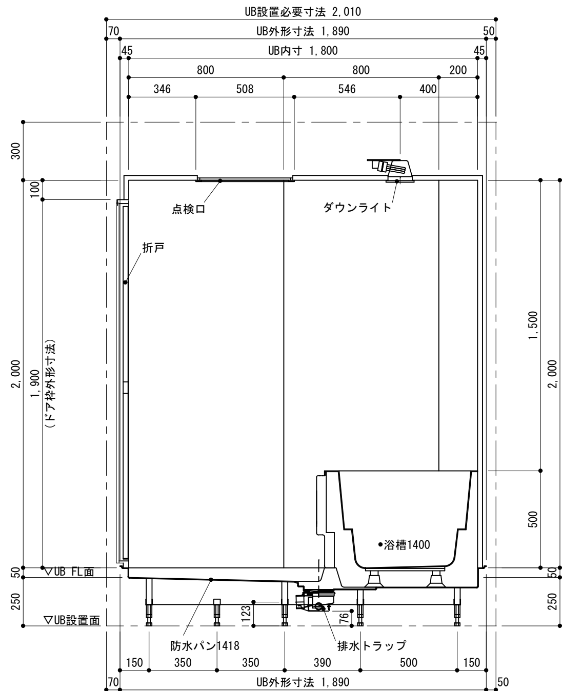
C展開図
