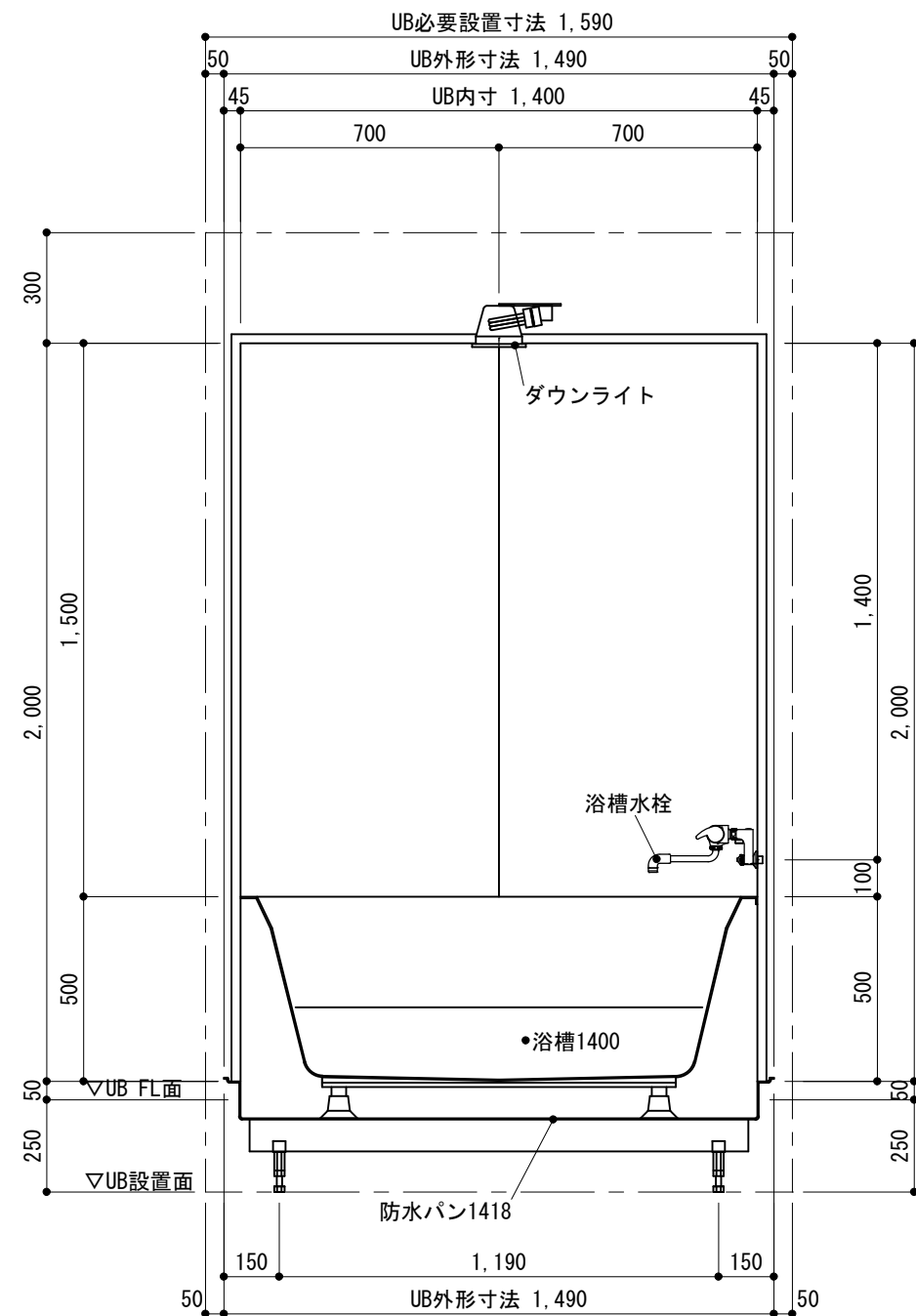
D展開図
