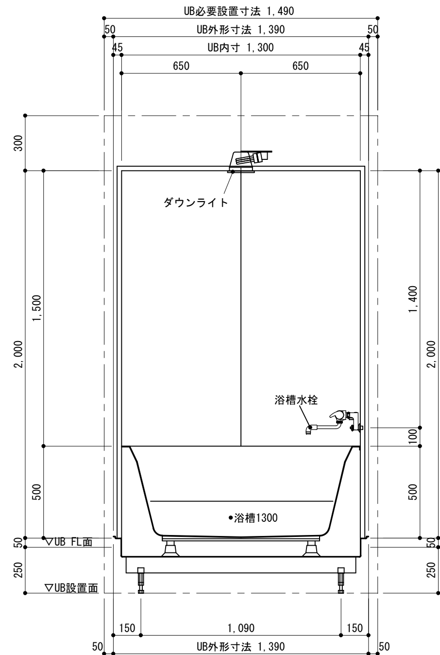
D展開図
