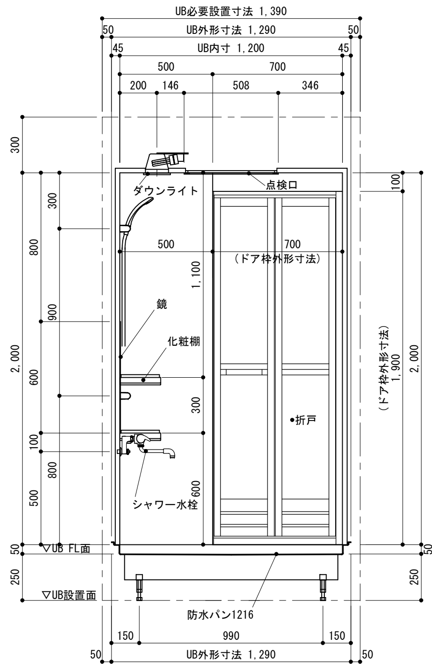
B展開図
