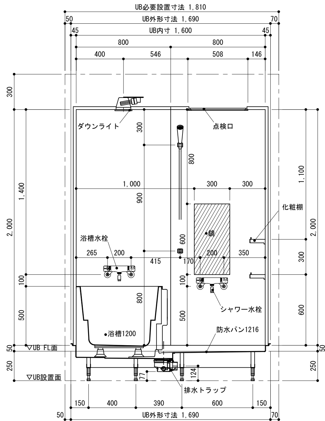
A展開図
