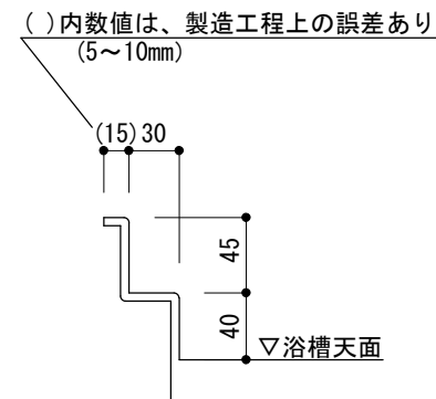
壁載り (防水リム) 部詳細 S=1/5
