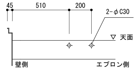
カウンター水栓 取付部詳細
