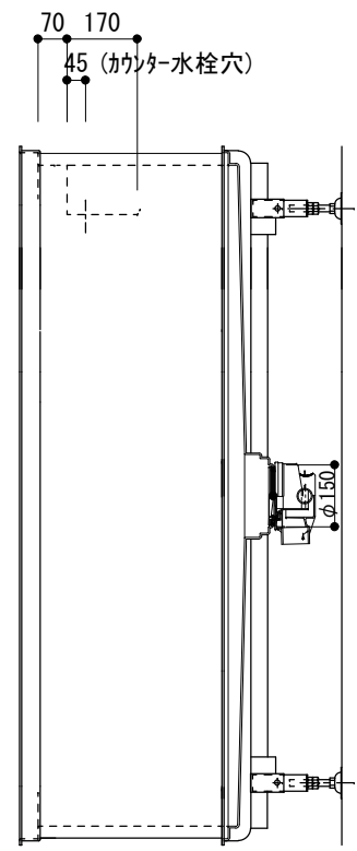
壁載り (防水リム) 部詳細 S=1/5
