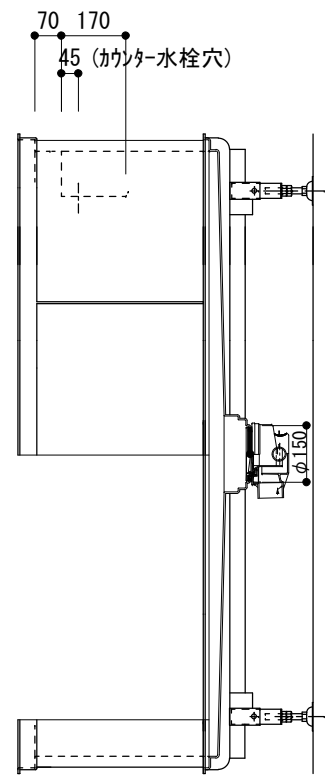
壁載り (防水リム) 部詳細
