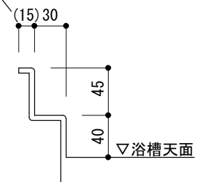
壁載り (防水リム) 部詳細
