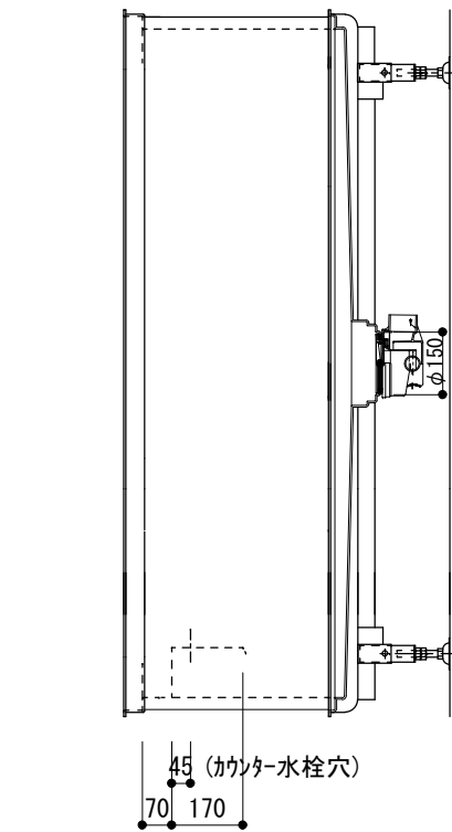
壁載り (防水リム) 部詳細 S=1/5
