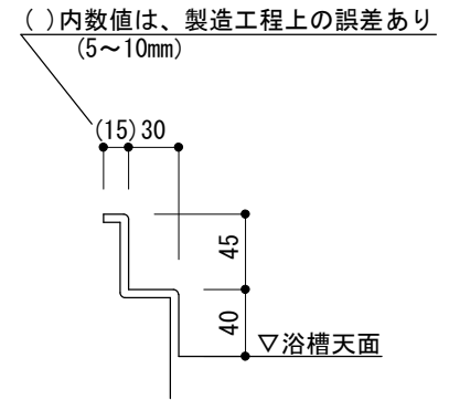
壁載り (防水リム) 部詳細 S=1/5
