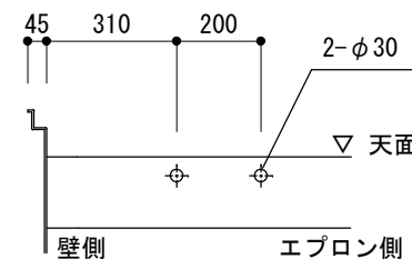
カウンター水栓 取付部詳細
