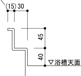
壁載り (防水リム) 部詳細 S=1/5
