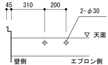
カウンター水栓 取付部詳細
