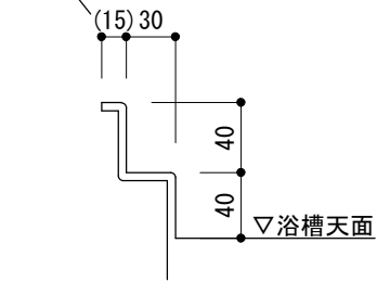
壁載り (防水リム) 部詳細 S=1/5
